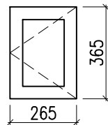
01 – SCHEMAT (SKALA 1:20)
