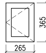
02 – SCHEMAT (SKALA 1:20)
